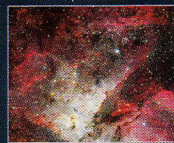
Gros plan sur la Carène
