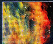
La nébuleuse de la Méduse
